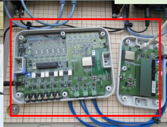
測定基板
